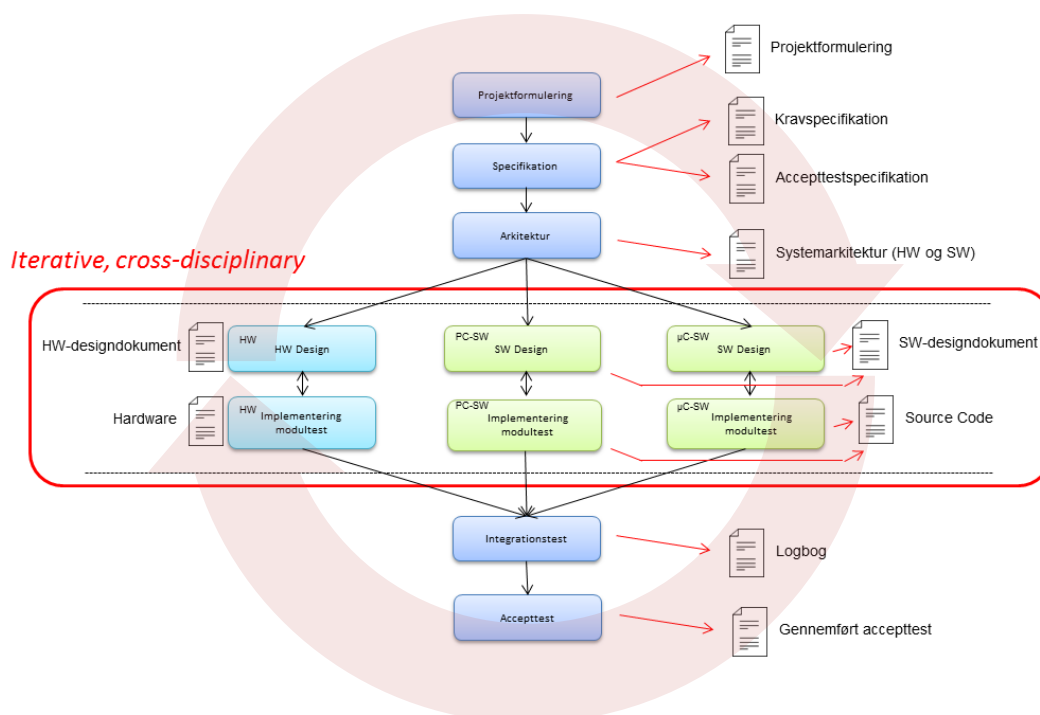
Figur 1 ASE-Modellen (Kilde: Kim Bjerge, Vejledning til udviklingsprocessen for projekt 2)
